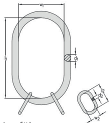
Ausführung Mehrstrang
